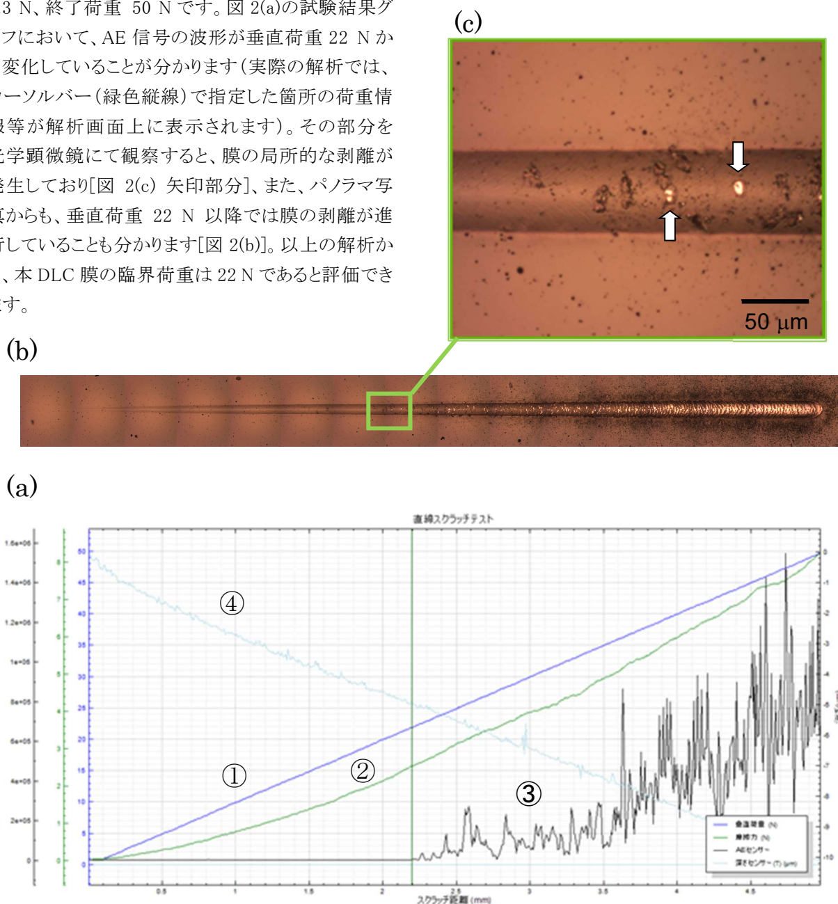
① 垂直荷重 (N), ② 摩擦力(N), ③ AE 信号, ④ 深さ(μm)
